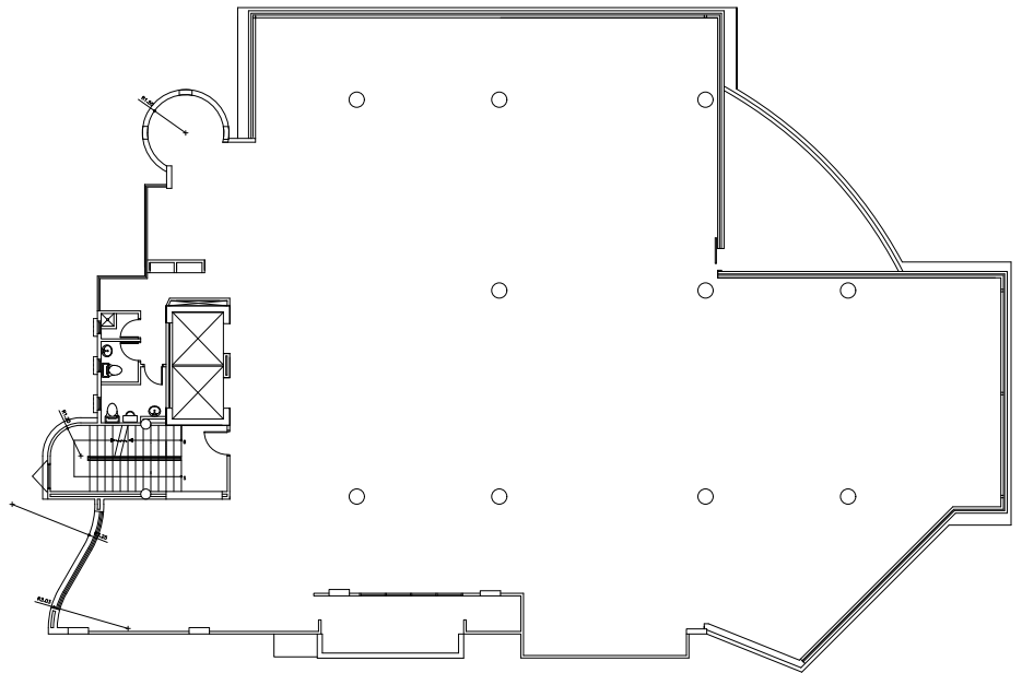
PLANTA ARQUITECTONICA - NIVEL 400 Esc. 1:50
