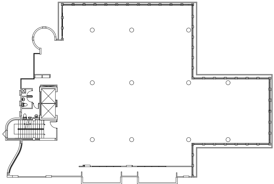
PLANTA ARQUITECTONICA_NIVEL 600 Esc. 1:50
