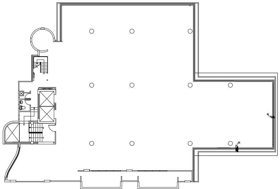
PLANTA ARQUITECTONICA NIVEL 700 ESC. 1:50
