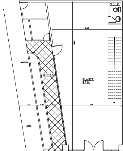
LOCAL 9 ESC. 1:100
