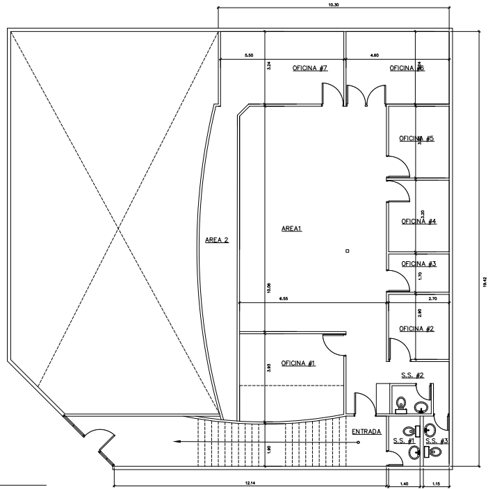
MEZZANINE ESC. 1:100
