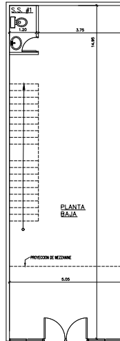
LOCAL 5 ESC. 1:100
