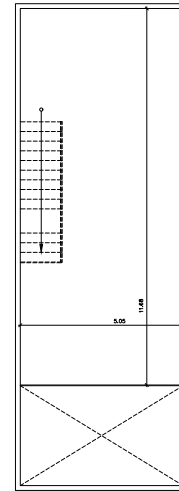
MEZZANINE ESC. 1:100
