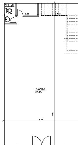
LOCAL 1 ESC. 1:100
