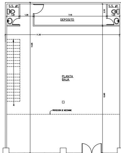
LOCAL 7-8 ESC. 1:100
