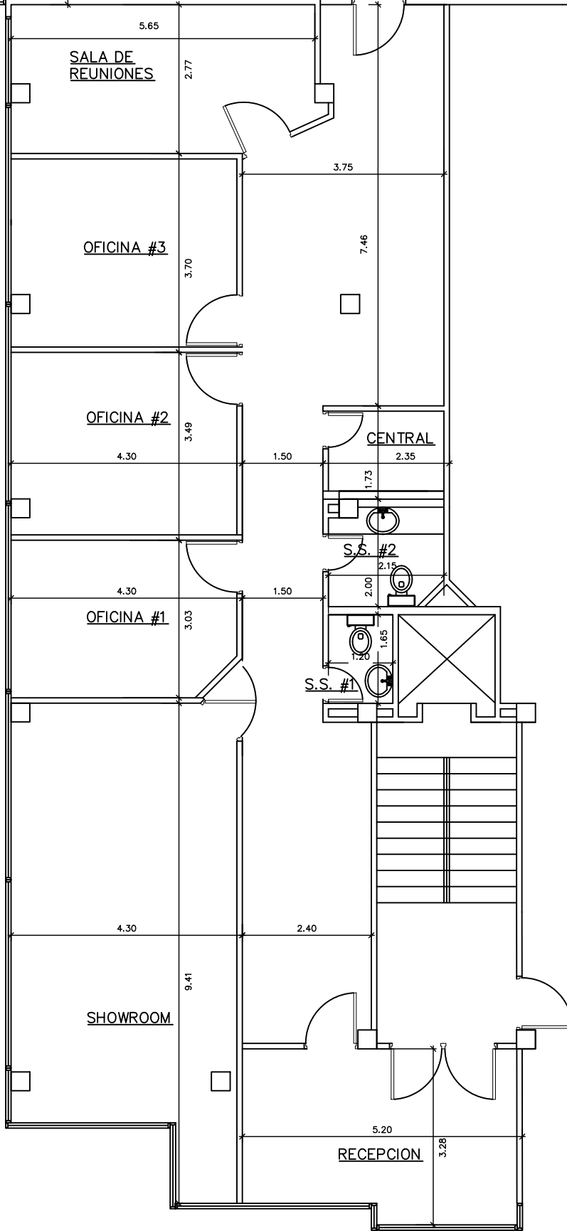
OFICINA 2-A ESC. 1:100
